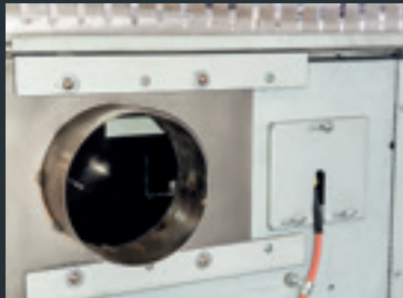
Uscita fumi posteriore regolabile fino a 7 cm Rauchrohranschluss bis zu 7 cm regulierbar
