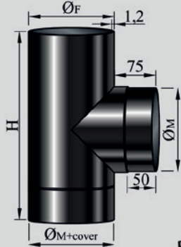
Te équerre avec tampon
