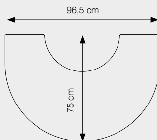
DEMI-CERCLE POUR DÉCOUPE DE VERRE POUR 7948 Réf.: 62928700
