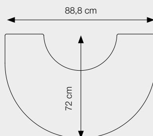
DEMI-CERCLE POUR DÉCOUPE DE VERRE POUR 7449 Réf.: 62928800
