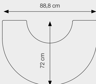
DEMI-CERCLE POUR DÉCOUPE DE VERRE (sauf 7349) Réf.: 62929400
